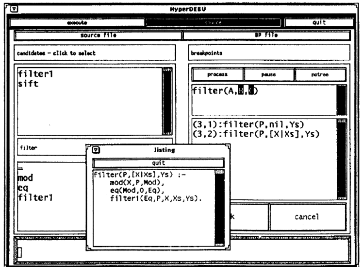
図3 データフローのブレークポイントの設定 Fig. 3 Setting breakpoints to visualize dataflow.
