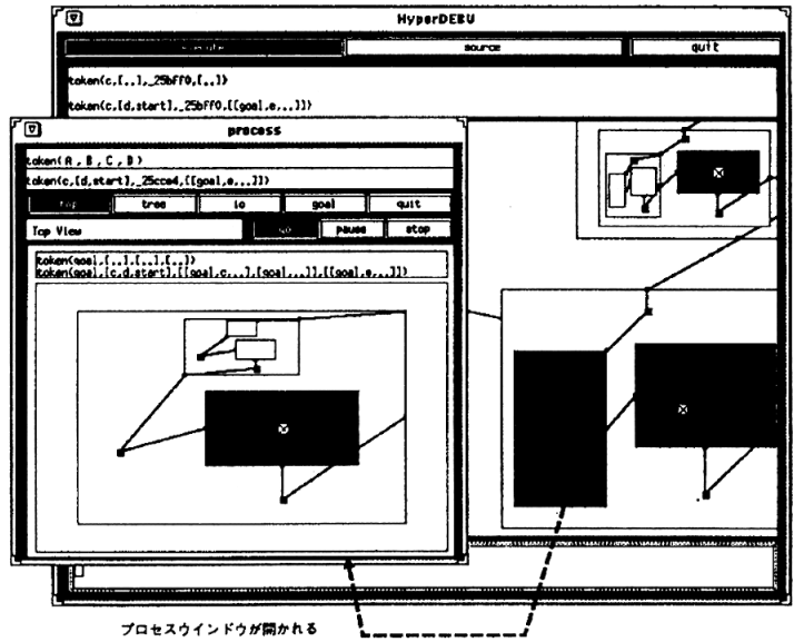
図 8 データフローの視覚化例 3—プロセスウインドウによる切りだし Fig. 8 Example of dataflow visualization 3.
