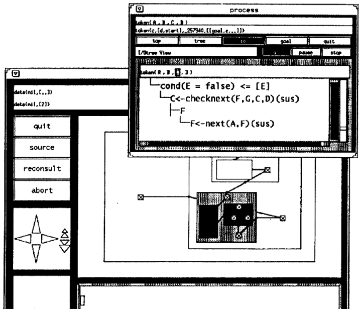
図 12 バグのあるプログラムの視覚化例 2
