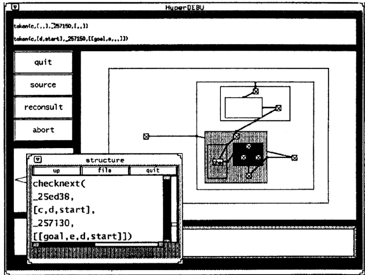
図 11 バグのあるプログラムの視覚化例 1
