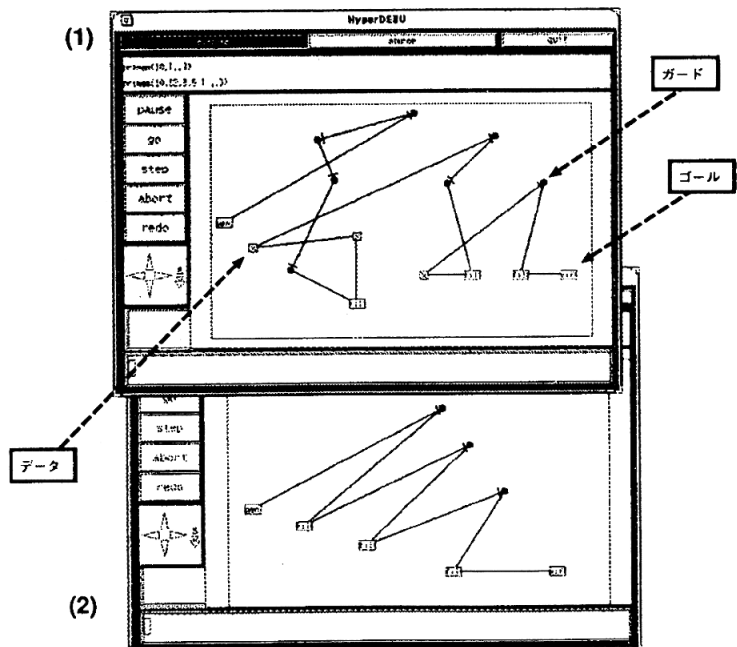
図6 データフローの視覚化例1 Fig. 6 Example of dataflow visualization 1.
