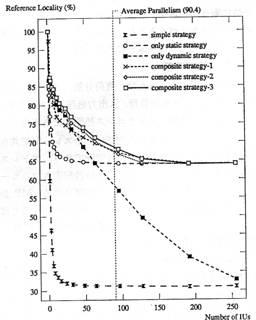
図7 IU台数の変化とローカルメモリ参照率 (6-Queen)
