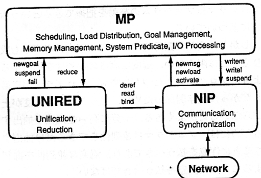
図 3 推論ユニット内の協調処理モデル Fig. 3 The cooperation model in Inference Unit.
