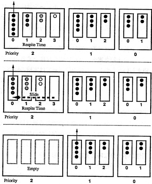
図 6 優先度ごとのスライド型レディーキュー Fig. 6 The sliding ready queue for each priority.
