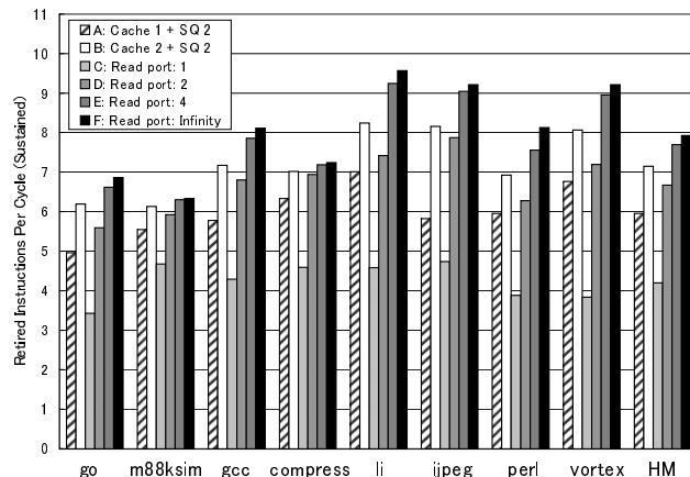
図 3: 拡張したストアキューによる性能向上
