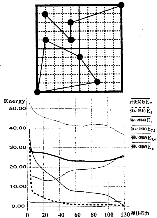
図7: 最適解へ収束なかった場合の解とエネルギー関数の値の変化
