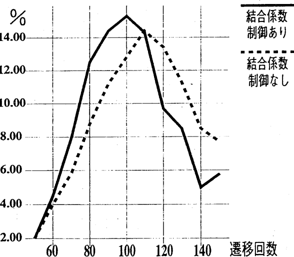
図8: エネルギー関数の結合係数の制御による収束速度改善
