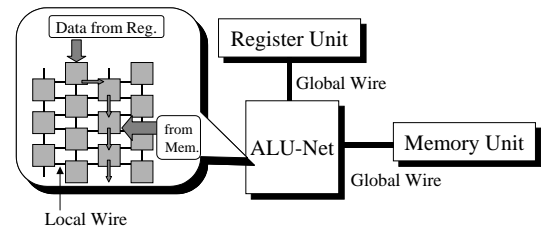
図 1: ALU-Net と Wire の構成
