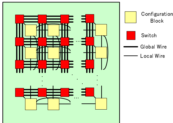
図 1: PD の内部
