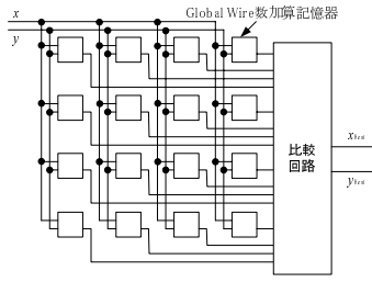
図 7: 使用 GW 数が少なくなるように CB 選択を行うハードウェア
