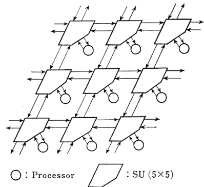
図 5 格子型網 Fig. 5 Mesh-connected network.
