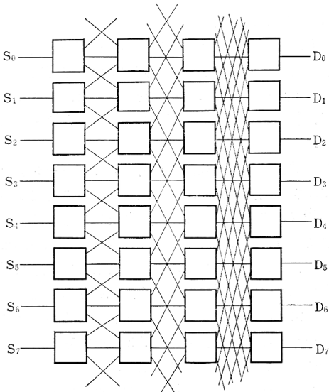
図6 ガンマ網 ( N=8 ) Fig. 6 Gamma network ( N=8 ).
