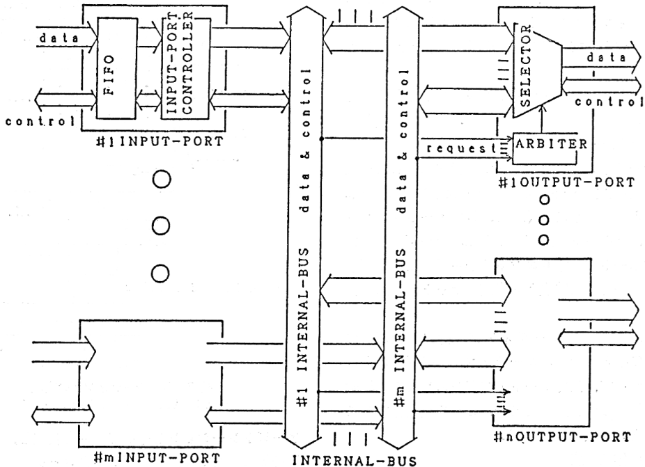
図1 SUの全体構成 Fig. 1 Overview of SU.
